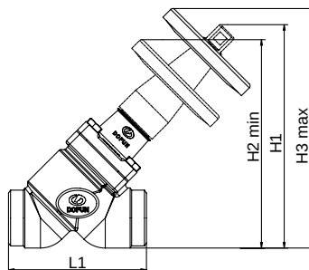
对接焊图示 BW
