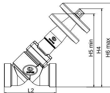
承插焊图示 SOC
