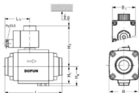
DEVS32 DEVS40 DEVS50结构示意图 DEVS32 DEVS40 DEVS50 Structure Diagram
