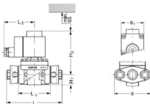
DEVS15 DEVS20结构示意图 DEVS15 DEVS20 Structure Diagram
