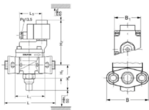
DEVS25结构示意图 DEVS25 Structure Diagram
